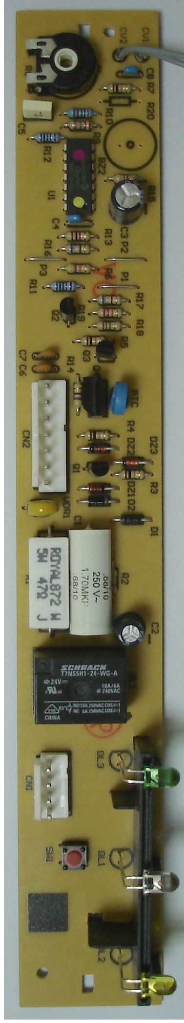
Плата управления холодильника ARDO CO 3012 SA. Вид со стороны компонентов
