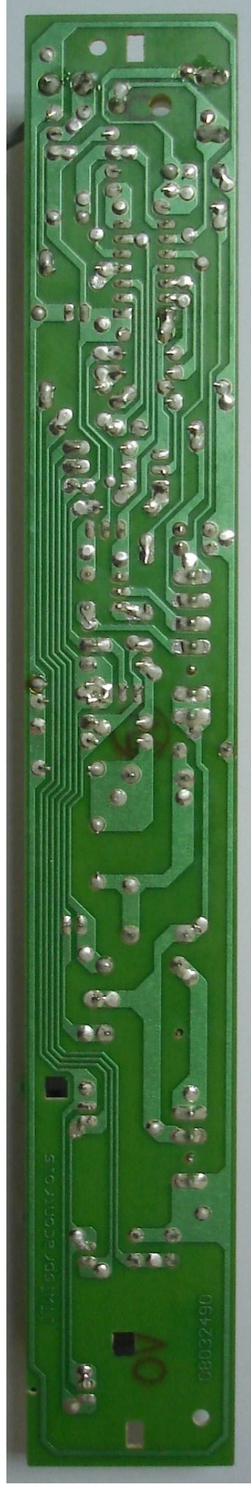
Плата управления холодильника ARDO CO 3012 SA. Вид со стороны монтажа, плата перевернута относительно горизонтальной оси.
