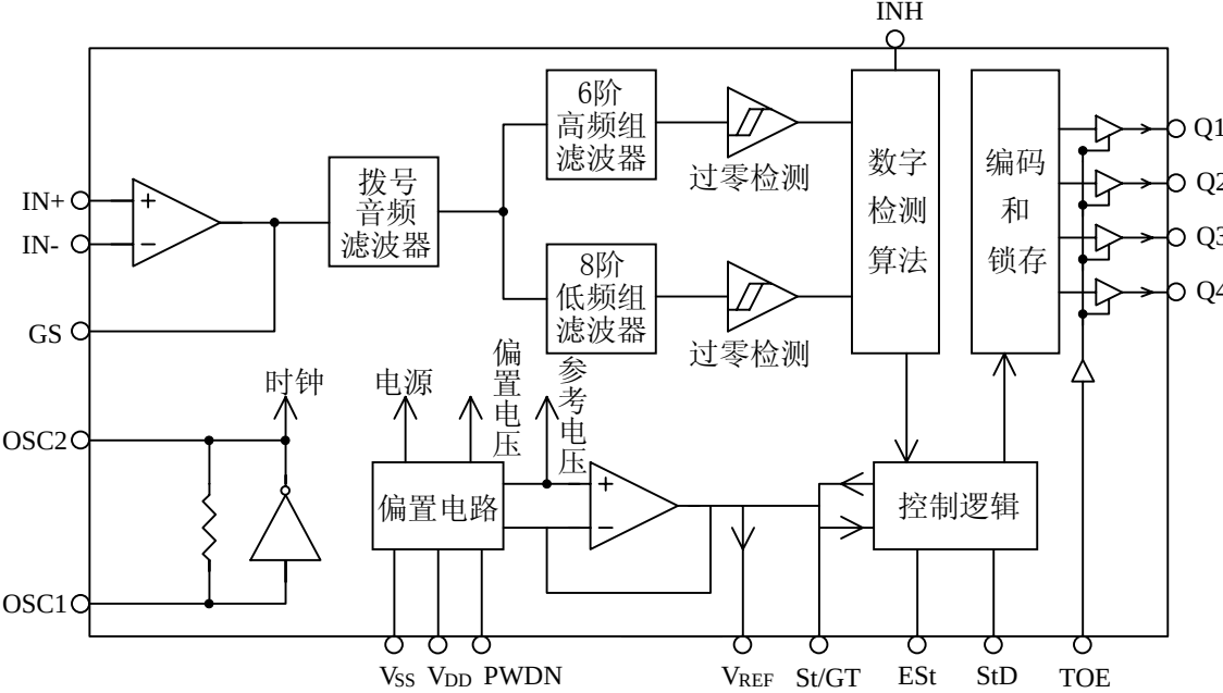
功能框图
