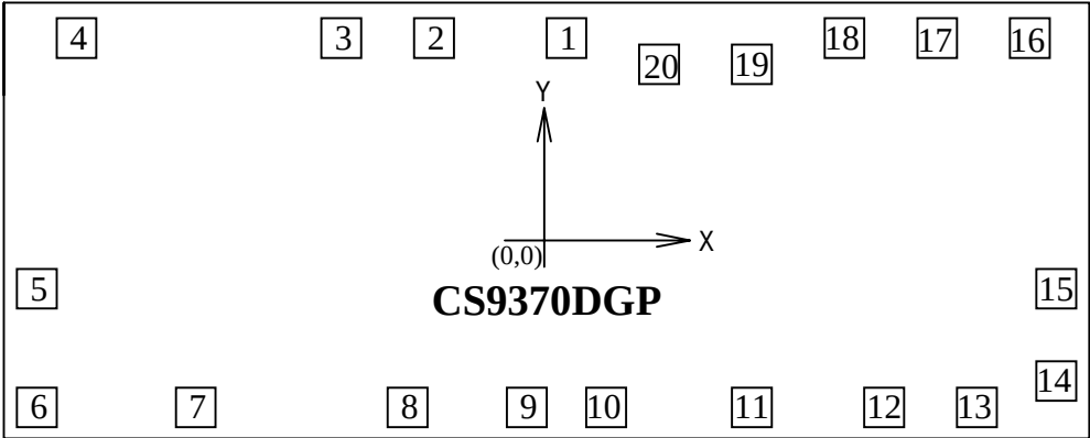
压焊点坐标
